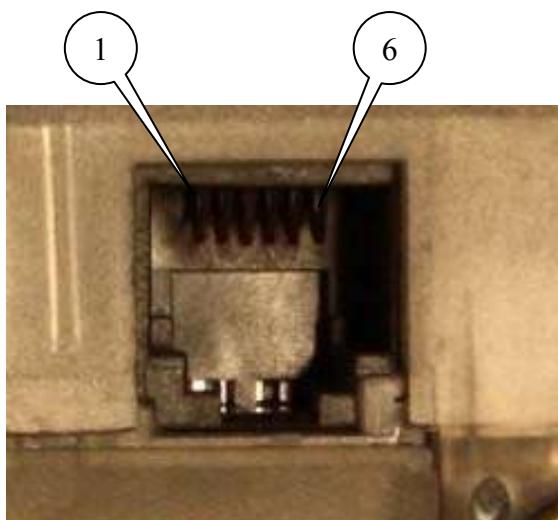
Рис.2.5.2 Разъём RJ11
