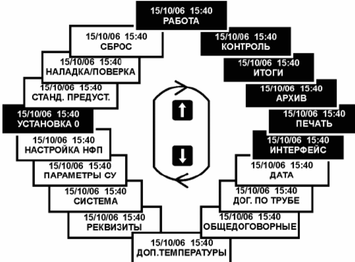
Рисунок 3 – Структура меню тепловычислителя ВКТ–5
