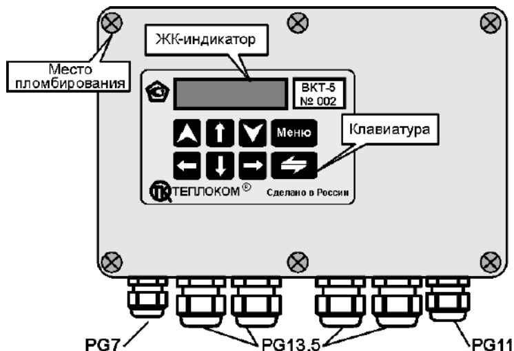
Рисунок 1 – Внешний вид вычислителя
